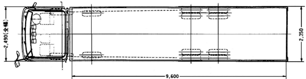
荷台図
