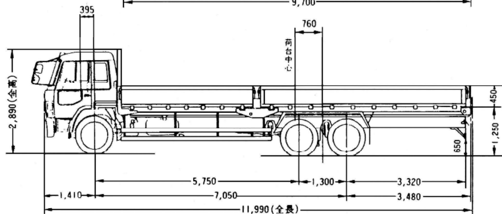
外観図
