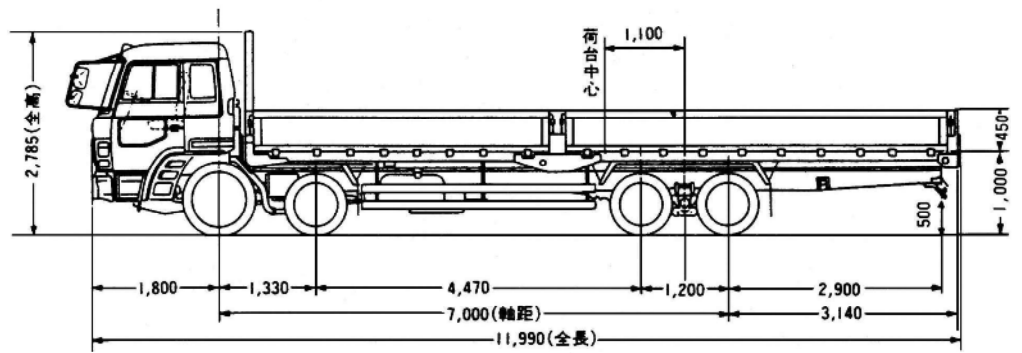
外観図
