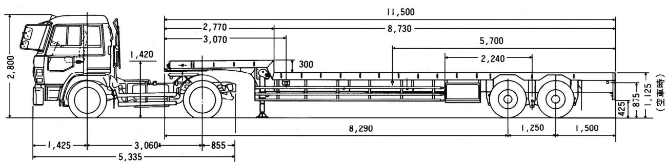
外観図
