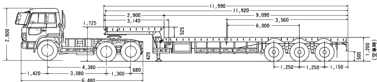
外観図
